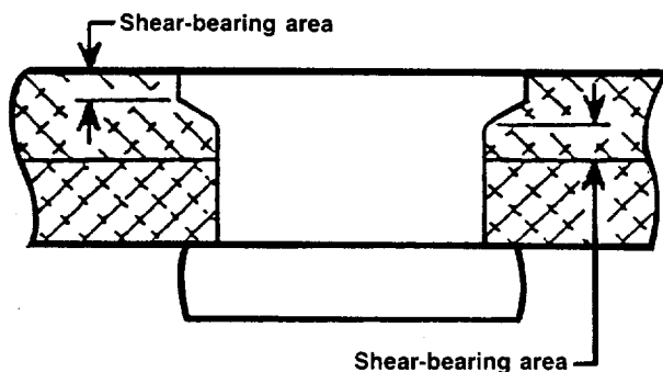
Figure 35.—BRZF 'fast' rivet.
